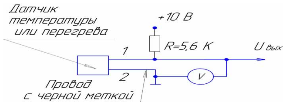
Рис.7 - Схема проверки датчика температуры или перегрева
