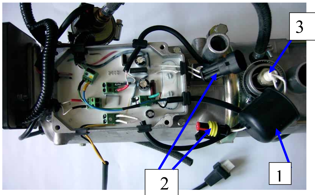
Рис.1 - Нагреватель (блок управления расположен в алюминиевом корпусе)
